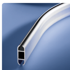
36.3445.31 Bogen 45° aus Schiene 2-Kanal FLACH Aluminium eloxiert R=250 mm mit gerade auslaufenden Enden Gesamtlänge=396 mm
